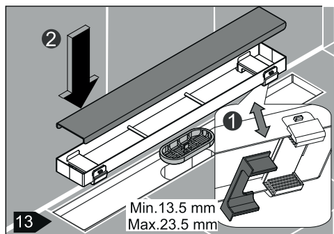
13. Регулировка высоты крышки
