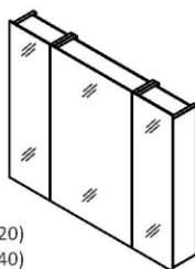
Зеркальный шкаф 800 (арт.071080) Зеркальный шкаф 200 (арт.071020) ШхВхГ- 1060x700x126
